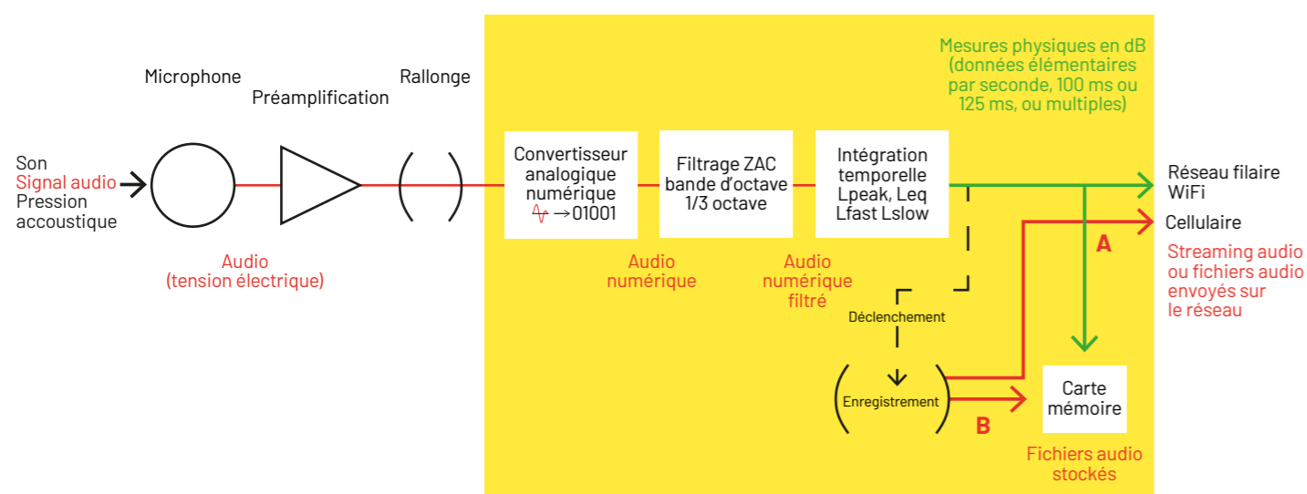
Schéma : Chaîne de traitement du son au sein d'un sonomètre
