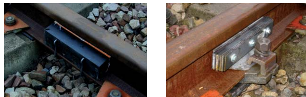
Exemples d'absorbeurs sur rail (Corus et Socitec)
